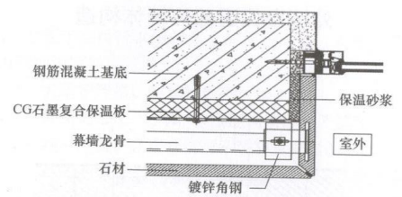
图 A.0.24 非透明幕墙窗侧口保温构造
