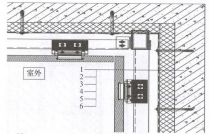
图 A.0.21 非透明幕墙阳角竖剖节点保温构造
