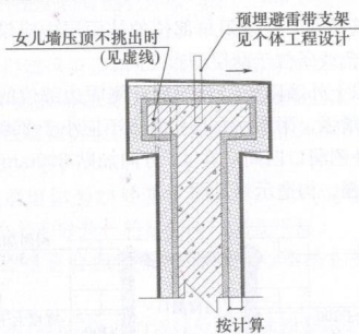
图 5.3.5 女儿墙部位构造示意
