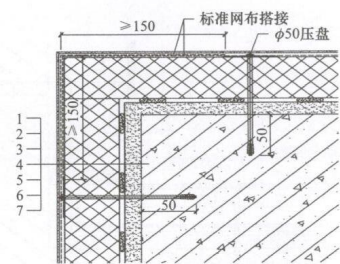
图 A.0.8 外墙阳角二层以上保温构造
