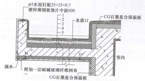
图 A.0.17 室外地坪以下垂直墙面有保温层的勒脚部位竖向剖面构造 1—防水；2—20厚1:3水泥砂浆找平；3—轻混凝土找纵坡；4—保温砂浆；5—钢筋混凝土基底。
