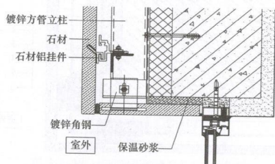
图 A.0.22 非透明幕墙窗上口保温构造
