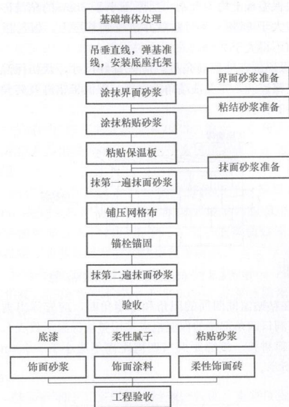
图 6.3.1 CG 石墨复合保温板外墙外保温系统施工工艺流程
