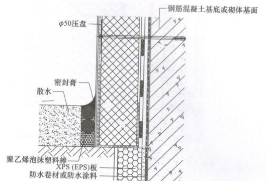
图 A.0.16 地下室外墙有保温层的勒脚部位竖向剖面构造
