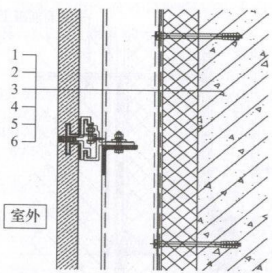
图 A.0.18 非透明幕墙竖剖节点保温构造
