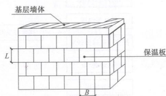
图 6.4.3-1 保温板错缝及转角铺贴示意
