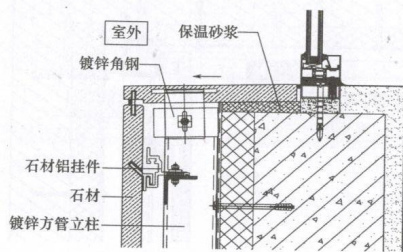
图 A.0.23 非透明幕墙窗台保温构造
