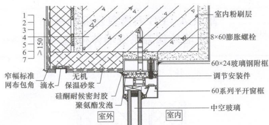
图 A.0.2 外墙窗上口剖面构造
