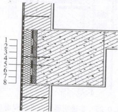
图 B.0.2 外墙自保温竖剖节点保温构造
