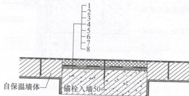
图 B.0.1 外墙自保温横剖节点保温构造
