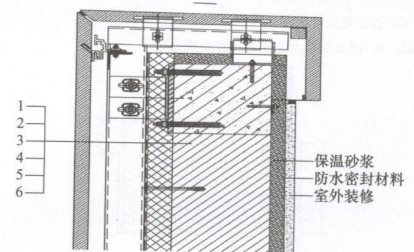
图 A.0.25 非透明幕墙女儿墙保温构造
