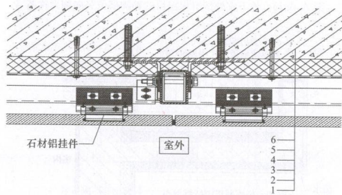
图 A.0.19 非透明幕墙横剖节点保温构造
