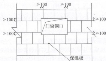
图 6.4.3-2 门窗洞口排版示意
