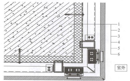
图 A.0.20 非透明幕墙阳角横剖节点保温构造
