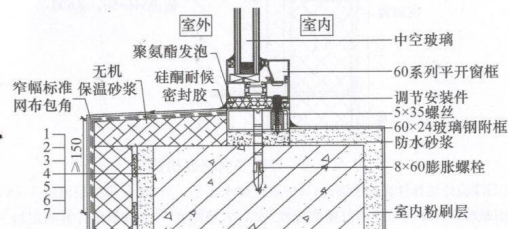
图 A.0.3 外墙窗下口剖面构造
